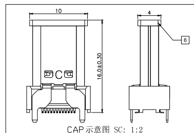
CAP 示意图 SC: 1:2
