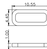
防水圈图示
