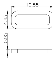
防水圈图示
