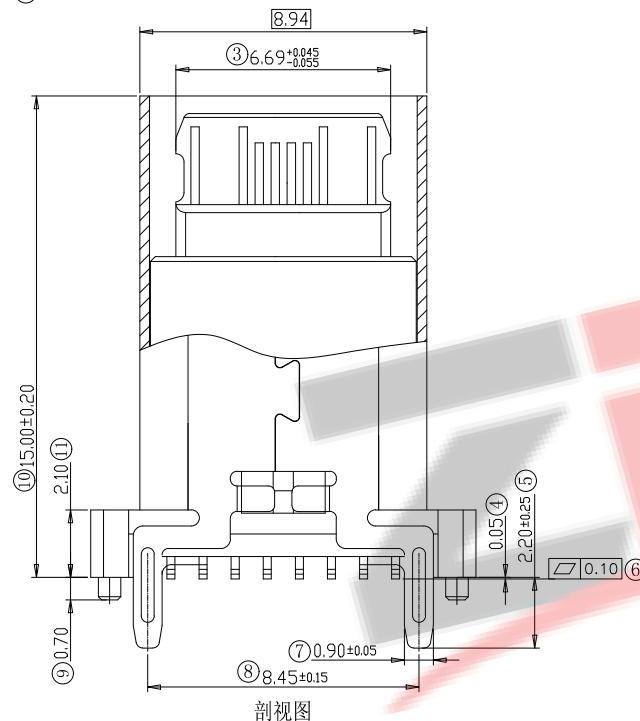
剖视图
