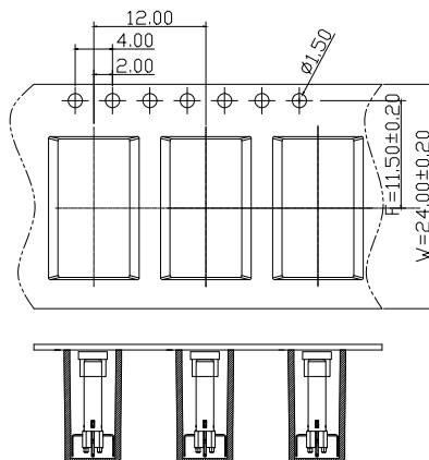
① 产品入载带示意图
