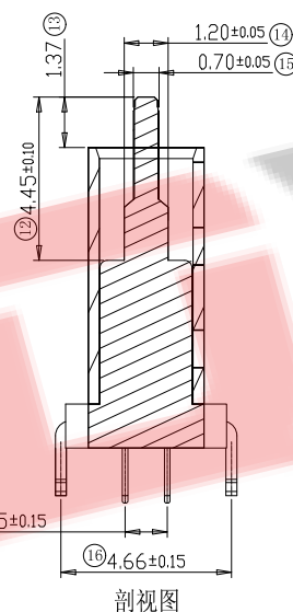
剖视图
