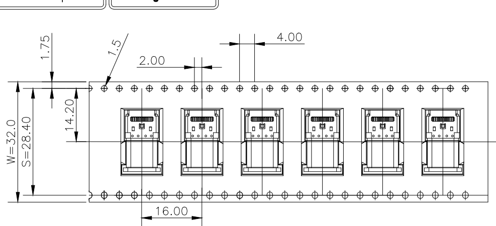
① 产品入载带示意图
