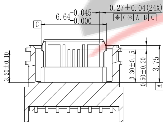
截面B-B
