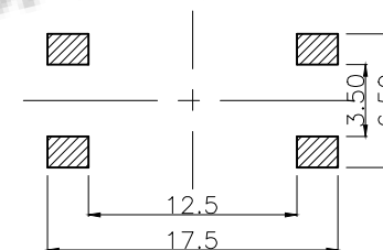
PCB. 焊接图
