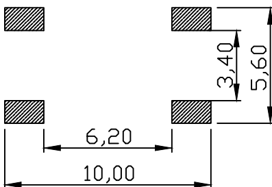
PCB. 焊接图
