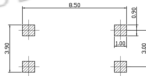
PCB. 焊接图
