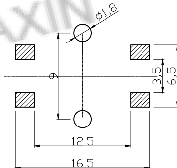
PCB. 焊接图
