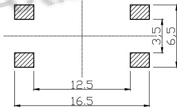
PCB. 焊接图
