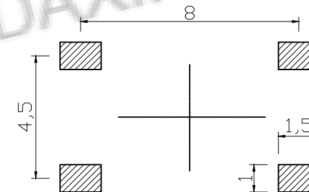
PCB. 焊接图
