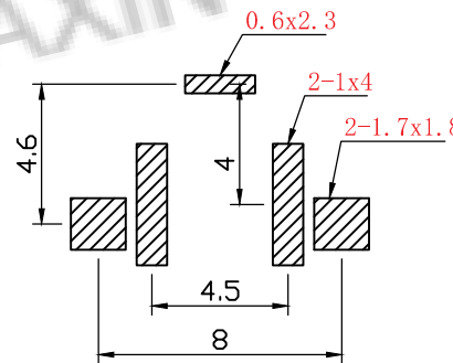
PCB. 焊接图
