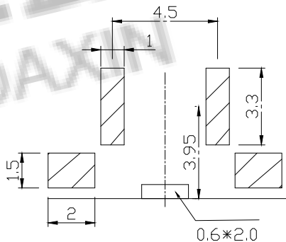
印制线路板图
