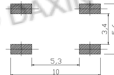
PCB. 焊接图
