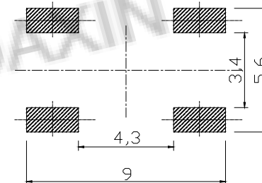
PCB. 焊接图
