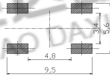
PCB. 焊接图
