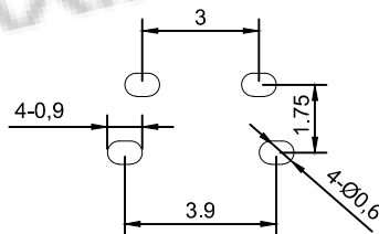
PCB. 焊接图
