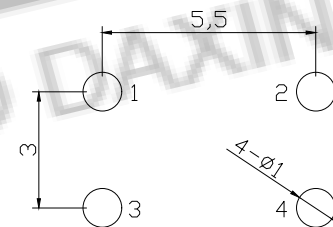
PCB. 焊接图
