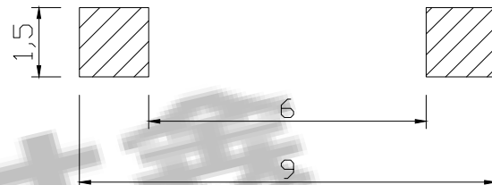
PCB. 焊接图
