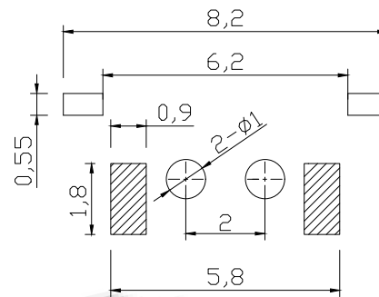
PCB. 焊接图
