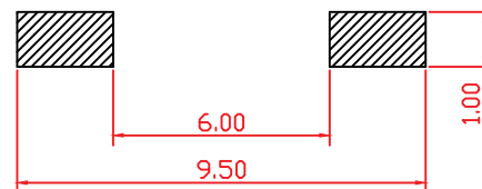
PCB. 焊接图
