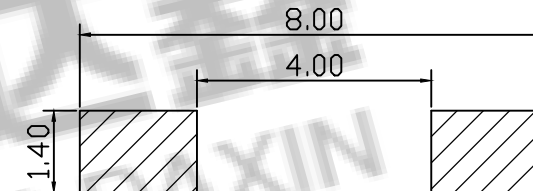
PCB. 焊接图
