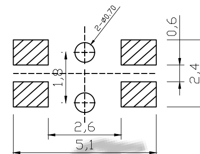
PCB. 焊接图
