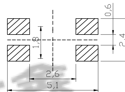
PCB. 焊接图
