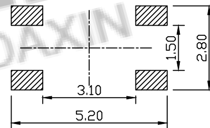
PCB. 焊接图
