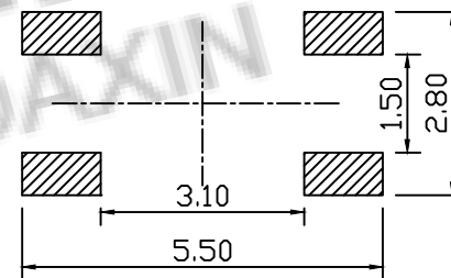
PCB. 焊接图
