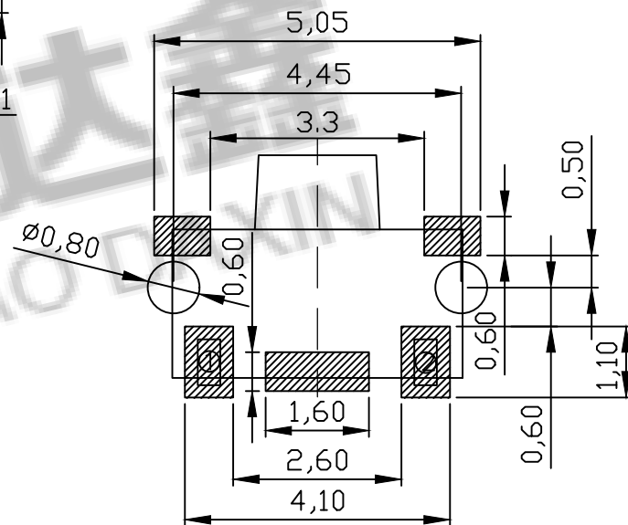
印制线路板开孔 P.C.B. HOLE DETAIL
