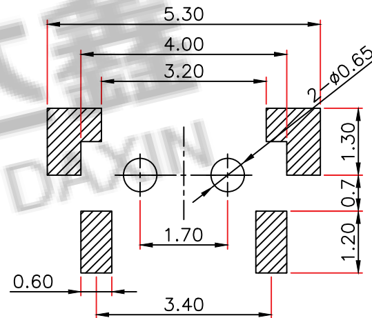
PCB. 焊接图
