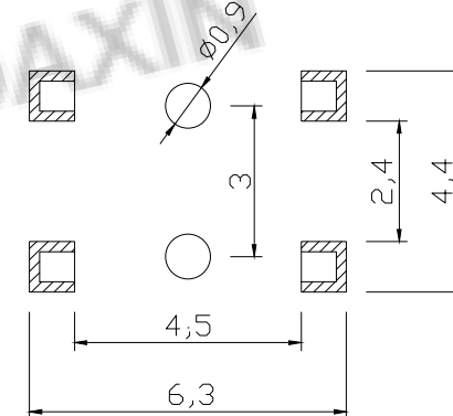
PCB. 焊接图
