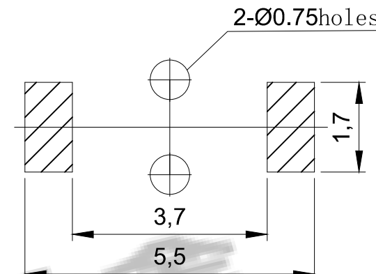
PCB. 焊接图
